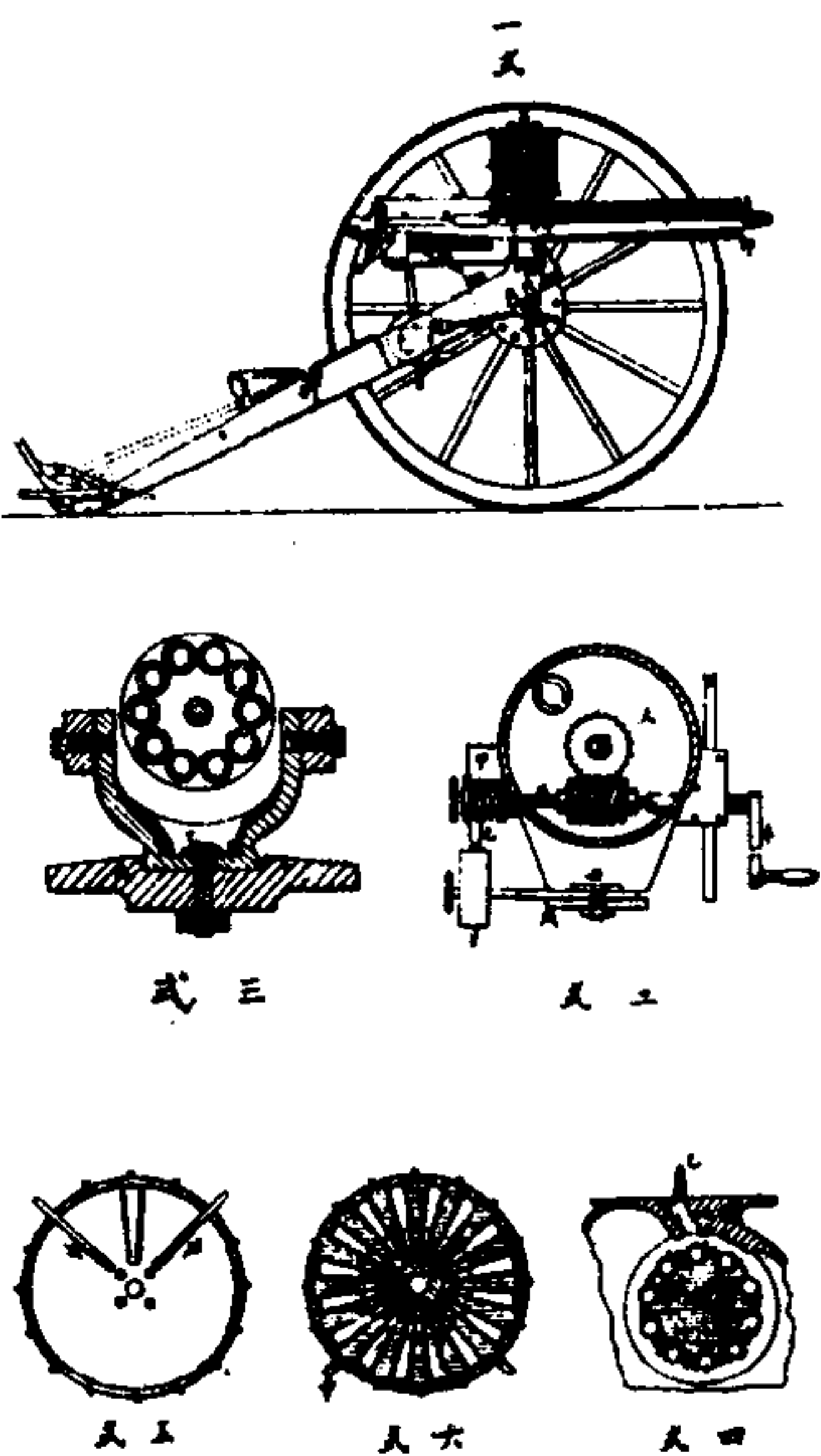
圖七十三百二第
