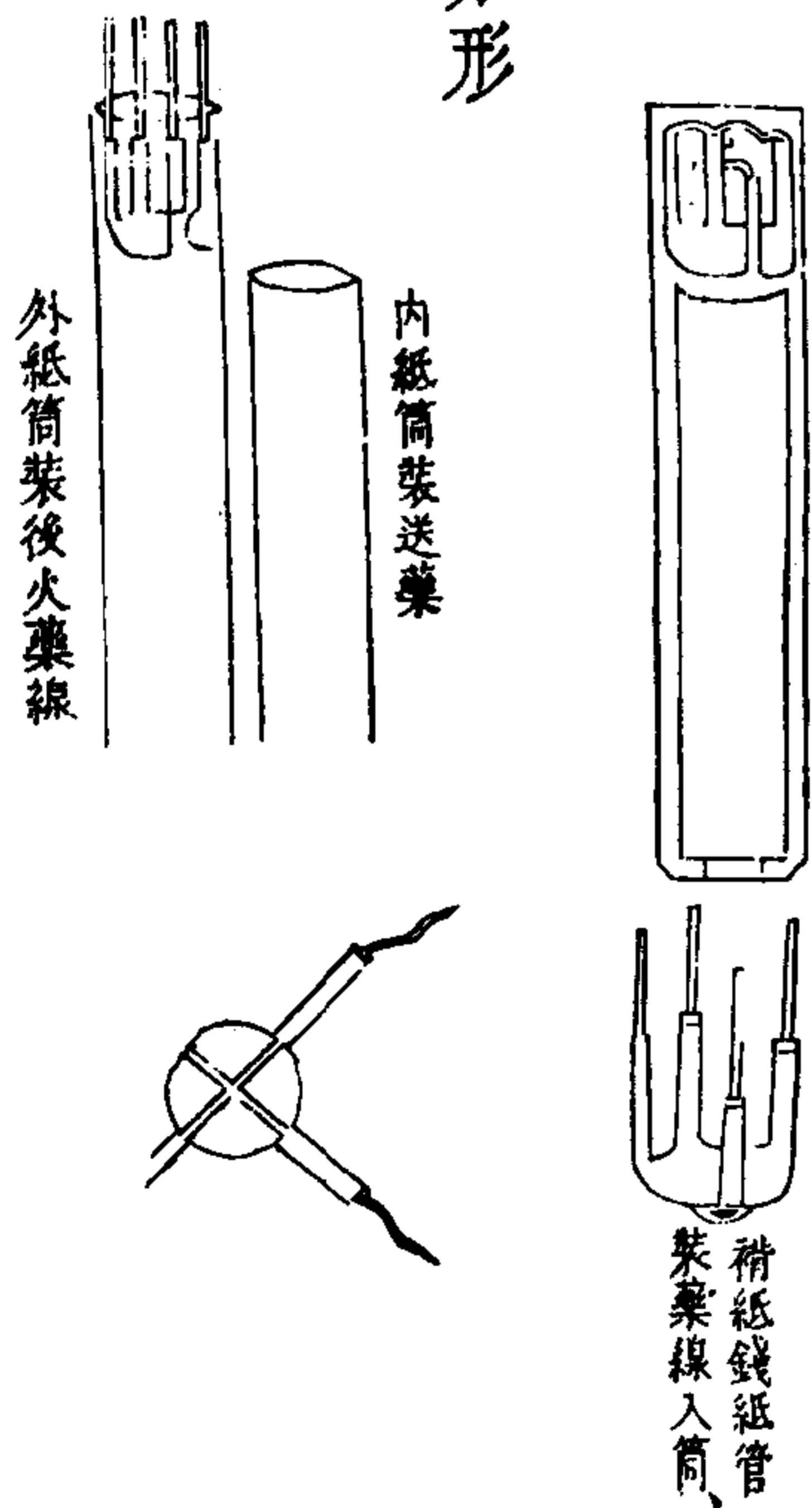
後火藥筒
