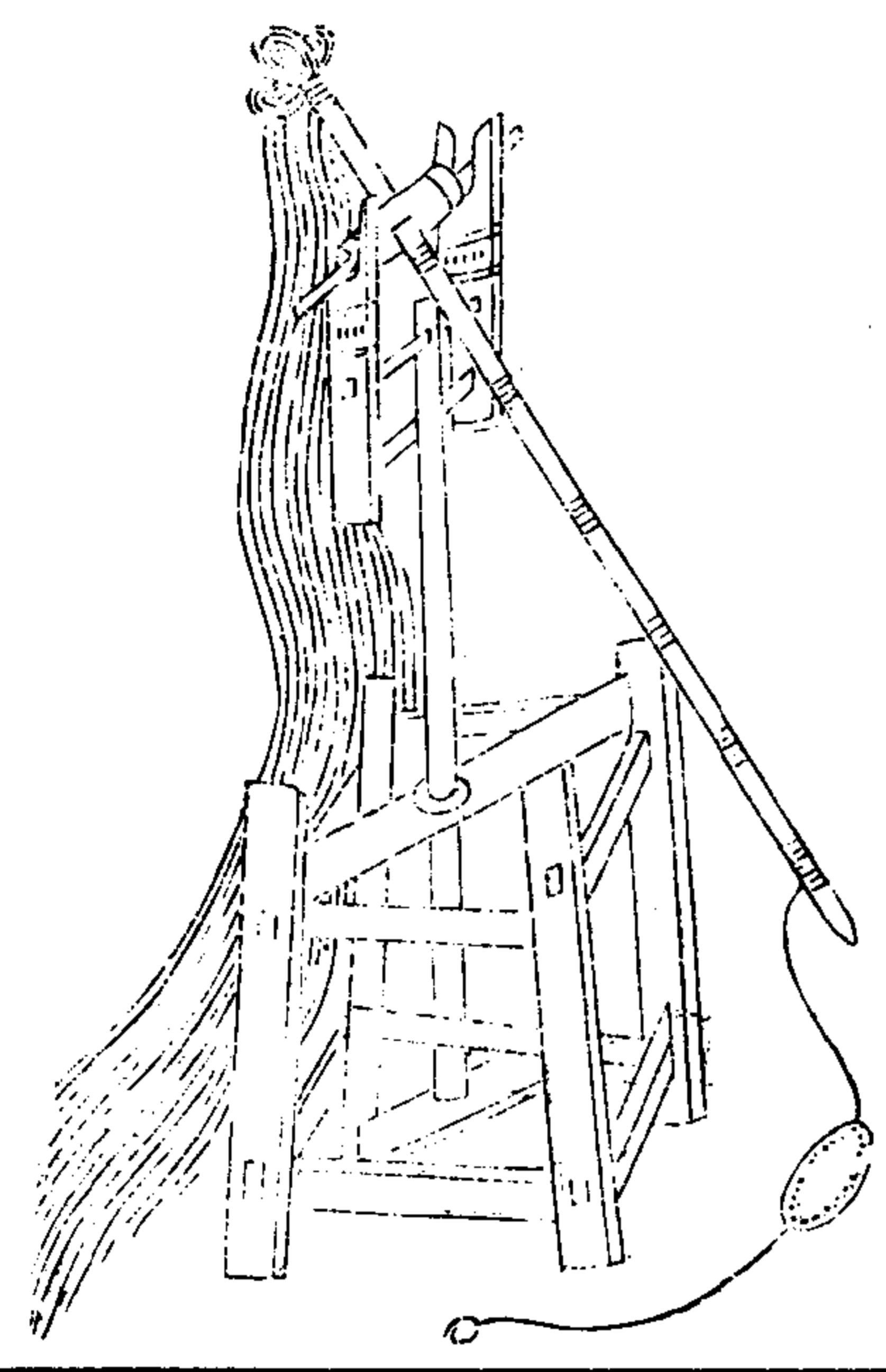
砲 風 旋 脚 獨
