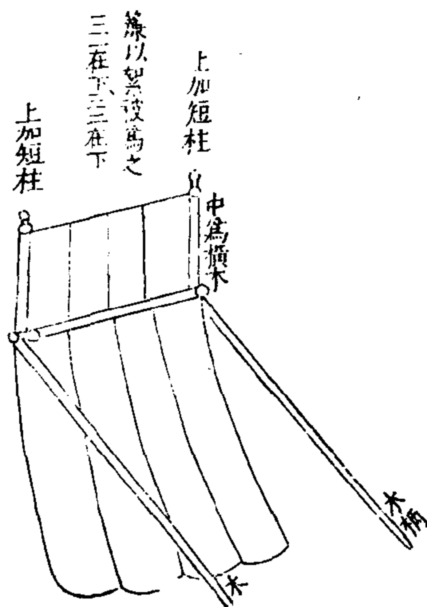
懸簾
