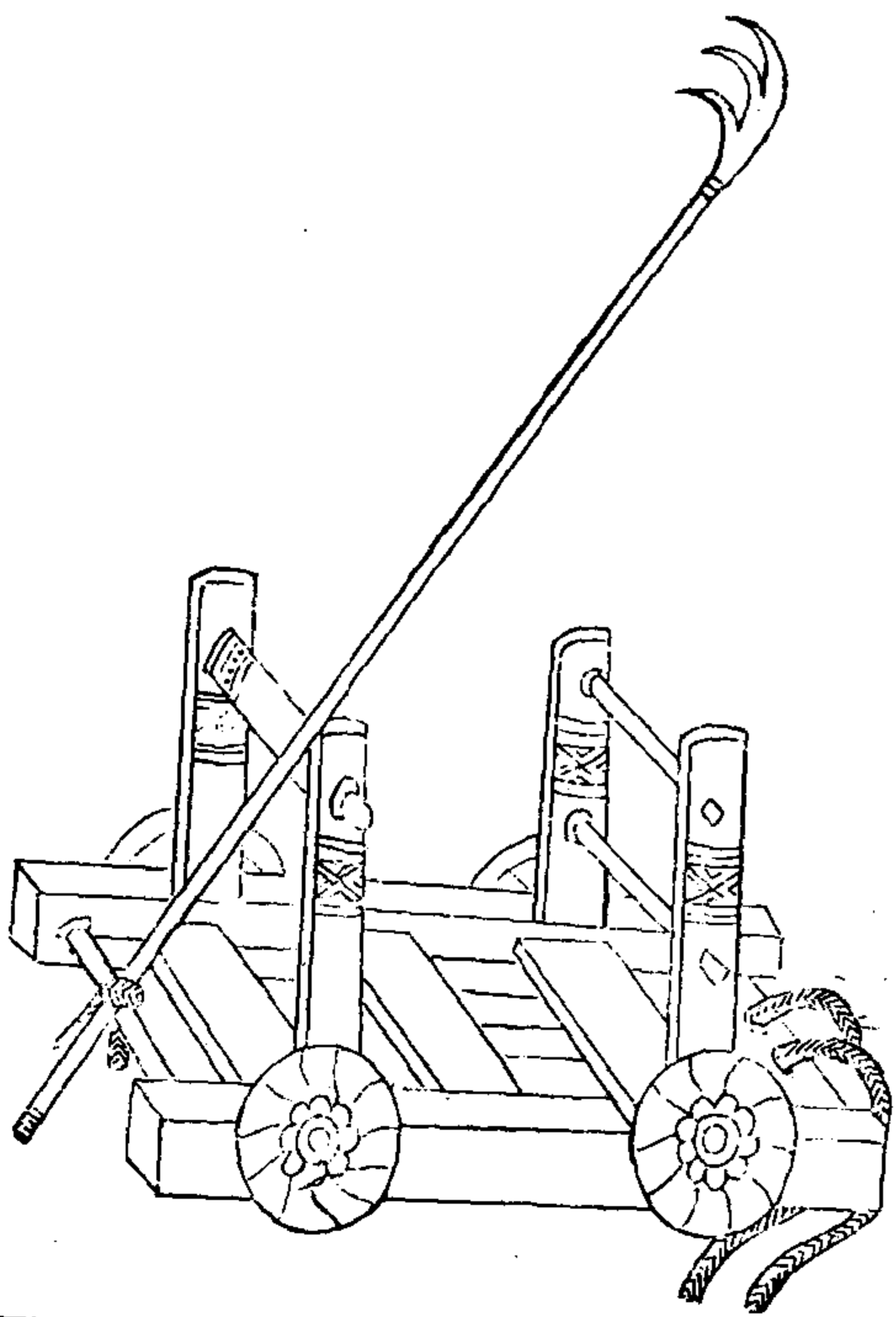
落車
