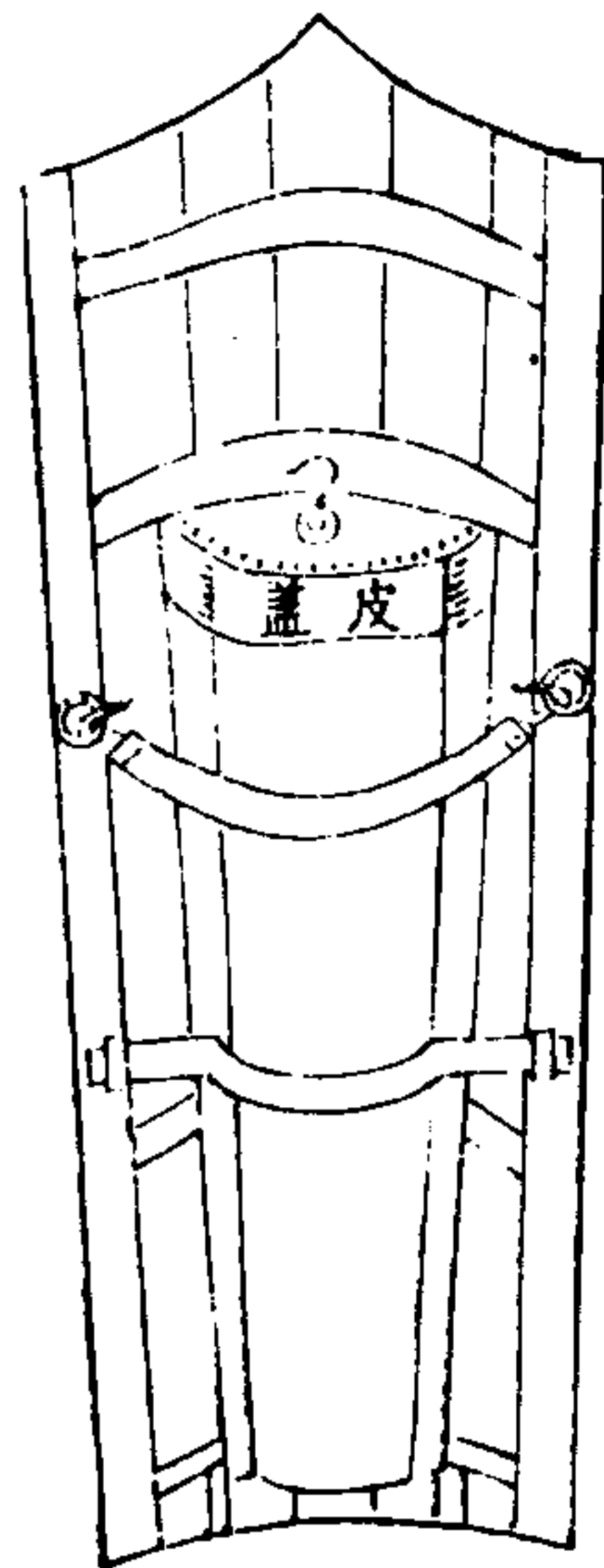
箭匣側形
