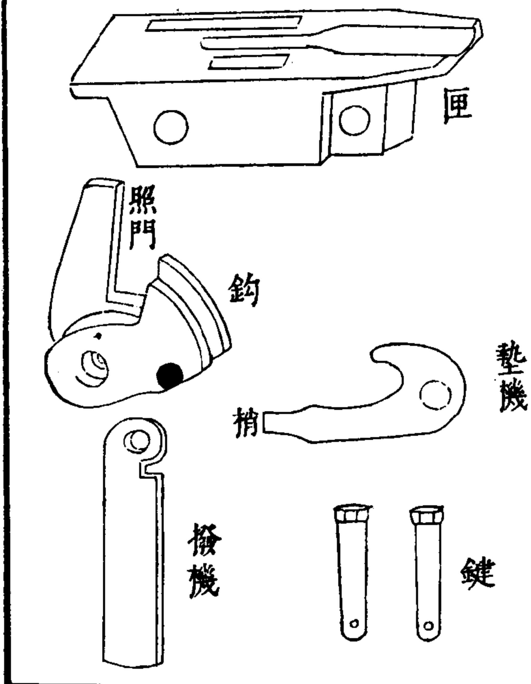
古銅弩機散圖
