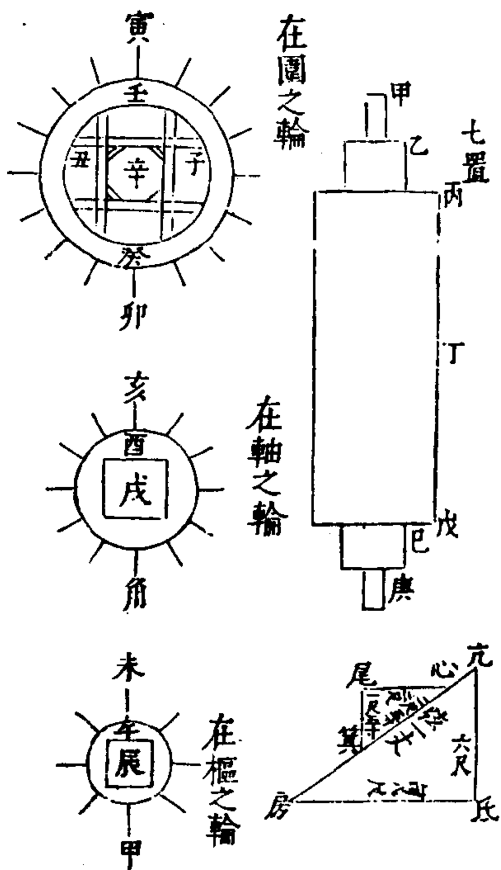
龍尾四圖
