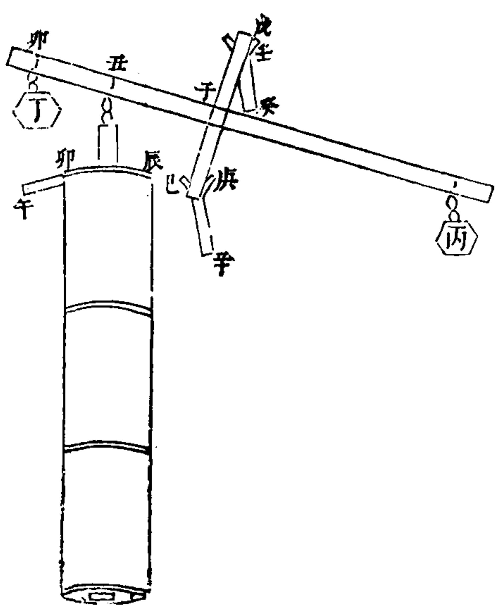
恒升三圖
