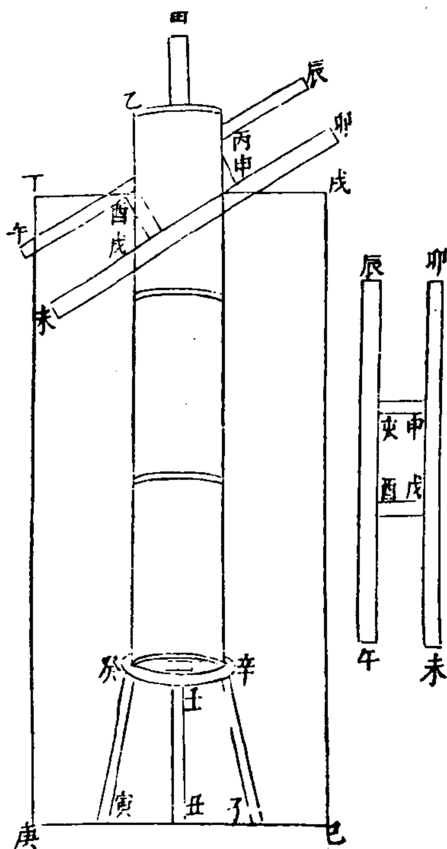
恒升四圖
